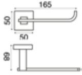
Kağıtlık (Kapaksız) Paper Holder (Without Cover) PL1020
