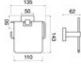
Kağıtlık Paper Holder PL1010
