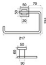
Yuvarlak Havluluk Towel Ring Siyah / Black PLB1083
