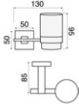
Diş Fırçalık Tumbler Holder PL1006
