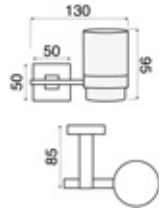
Diş Fırçalık Tumbler Holder Siyah / Black PLB1086
