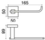
Kağıtlık (Kapaksız) Paper Holder (Without Cover) Siyah / Black PLB1090
