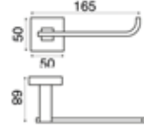
Kağıtlık (Kapaksız) Paper Holder (Without Cover) Mat Bronz / Mat Bronze PLM1060
