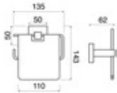
Kağıtlık Paper Holder Siyah / Black PLB1080
