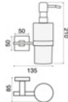
Sıvı Sabunluk Liquid Soap Holder Siyah / Black PLB1084A
